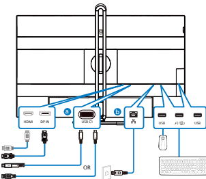
USB hub (USB A-C)
